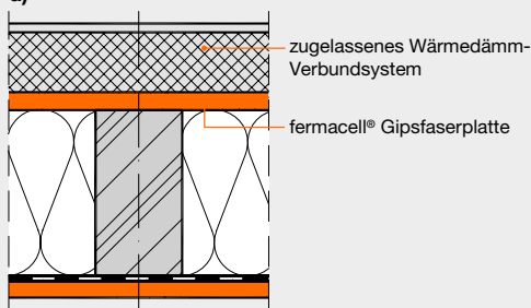
Wirksamer Wetterschutz WDVS
