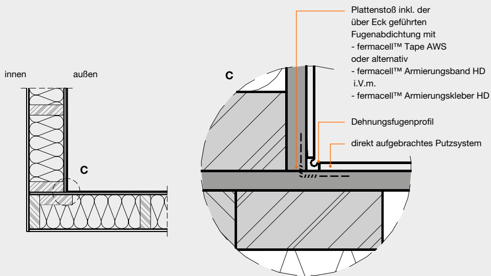
Ausbildung einer Innenecke im Außenwandbereich mit fermacell® Powerpanel HD
