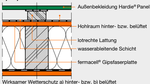
Wirksamer Wetterschutz a) hinter- bzw. b) belüftet
