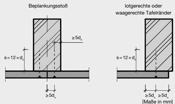
Bild 5: Erforderliche Randabstände für Nägel
