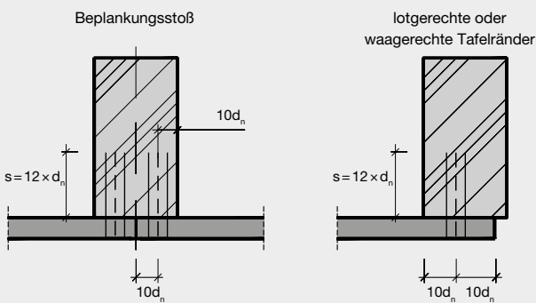
Bild 4: Erforderliche Randabstände für Klammern
