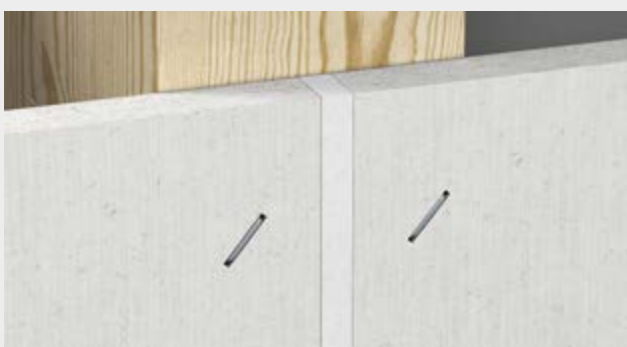
Spachtelfuge -Fugenbreite in Abhängigkeit der Plattendicke (s.a. Seite 137)
