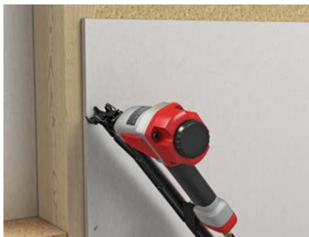
Abstand und Verbrauch von Befestigungsmitteln bei nichttragenden Wände pro m 2 mit fermacell® Gipsfaserplatten
