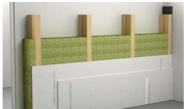
10 HT 21-205 fermacell™ Holzständerwand
