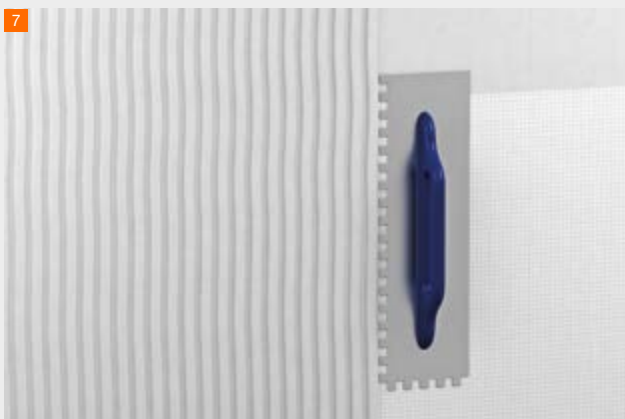
Eindrücken des fermacell™ Armierungsgewebes HD in das Mörtelbett
