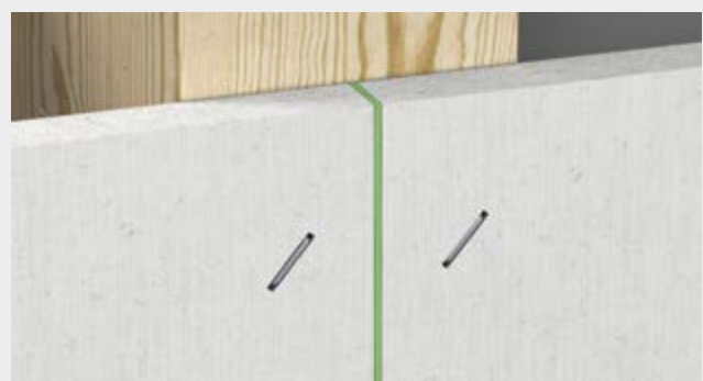
Klebefuge -Fugenbreite ≤ 1 mm
