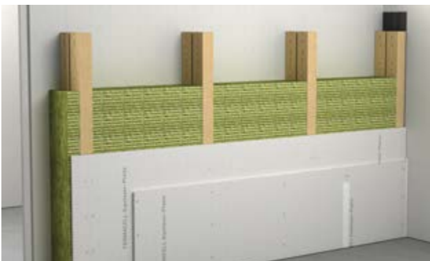
10 HT 31-405 fermacell™ Holzständerwand ■ abweichend feuerbeständig
