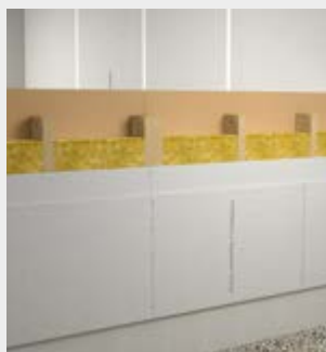
Abb. 6: Wandelementstoß – Vertikalfuge
