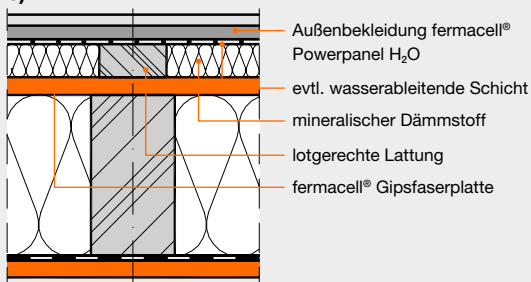
Dauerhaft wirksamer Wetterschutz nicht belüftet
