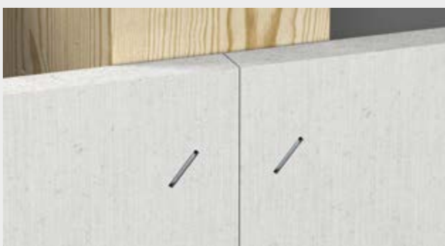
Plattenstoß dicht gestoßen -Fugenbreite ≤ 1 mm
