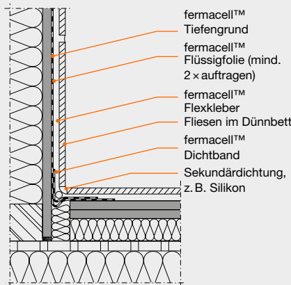
Boden-Wand-Anschluss
