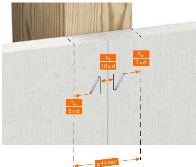
Verbindungsmittelabstand \geq 30^\circ
